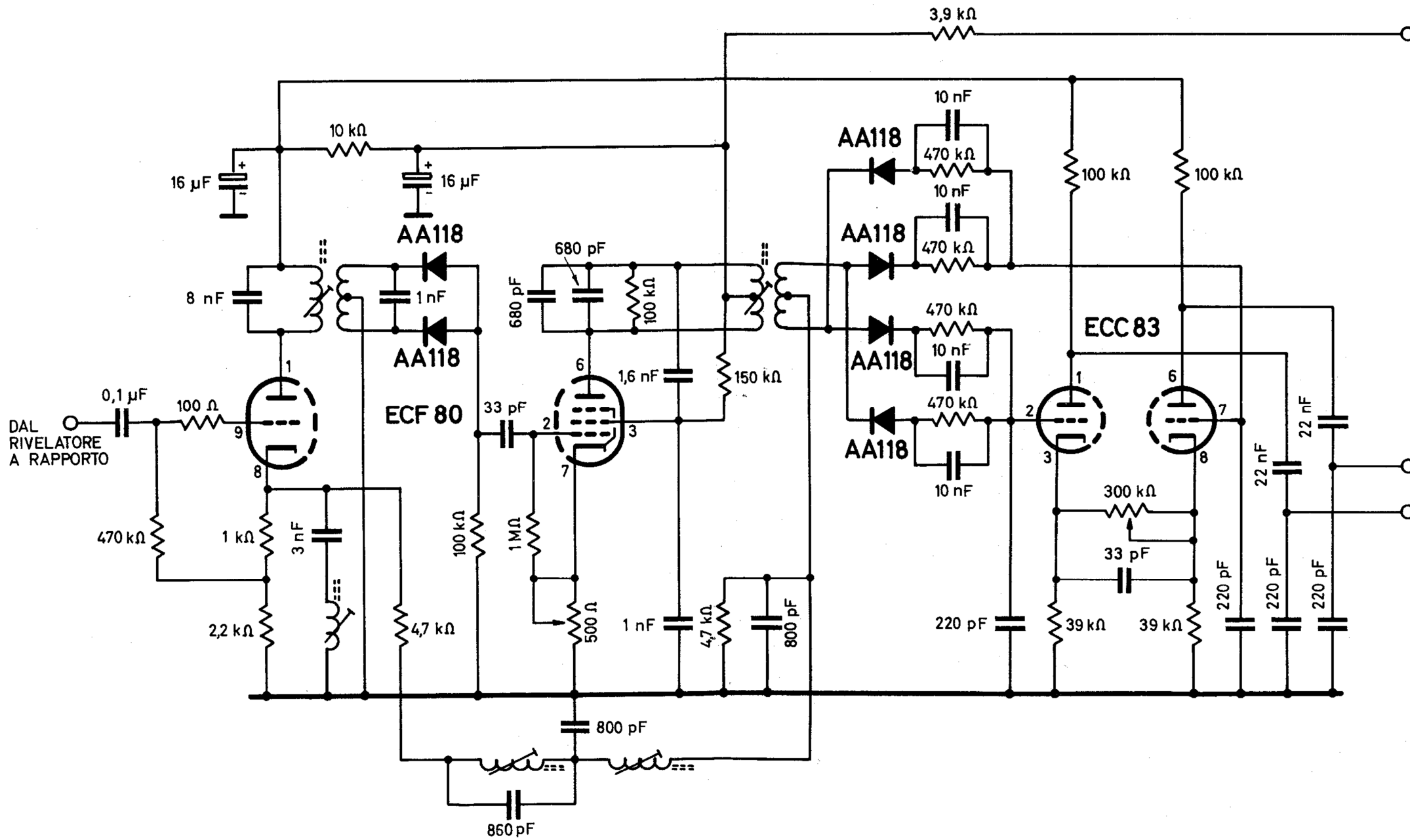
DECODER SIEMENS Mod. RE4210
